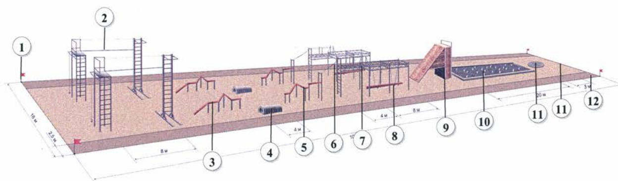
Рис. 48. Схема горной полосы препятствий
