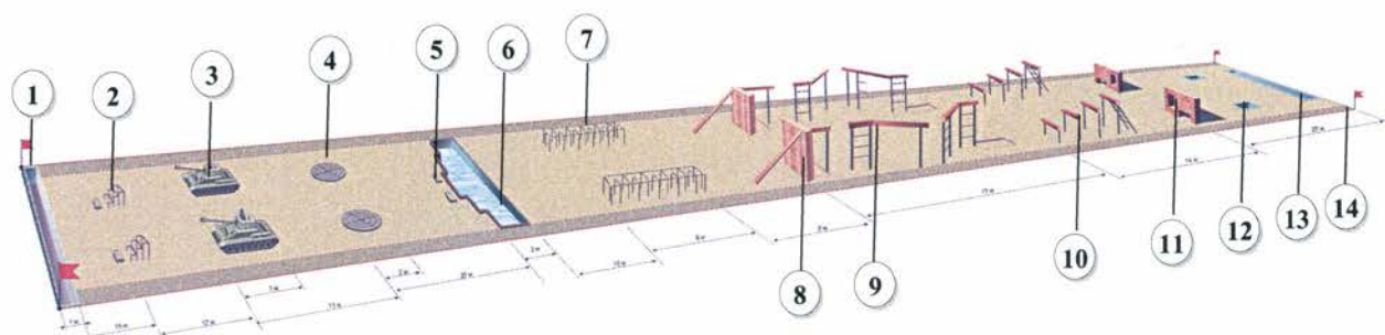
Рис. 45. Схема танковой полосы препятствий
