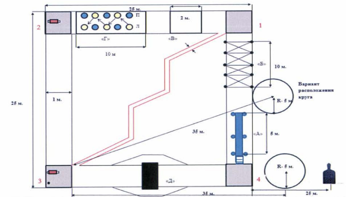
Рис. 91. Схема комплексного упражнения «Квадрат»
