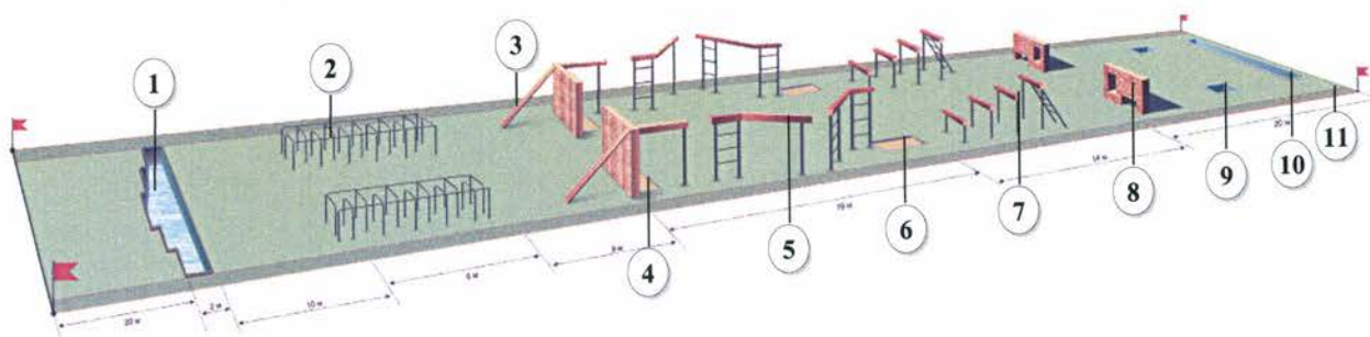
Рис. 43. Схема единой полосы препятствий
